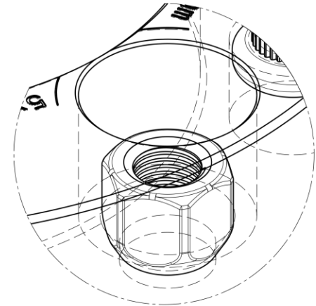
Detail A[2] Scale: 2:1
